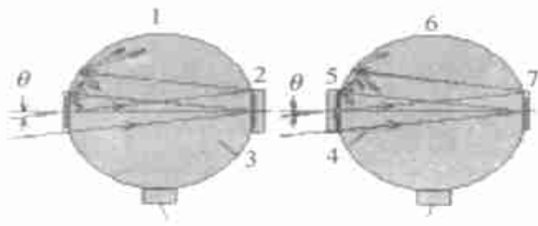
图 3 测量生物组织的镜面反射率和准直透射率的方法
