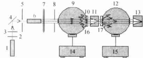
图 2 测量生物组织光学特性的双积分球系统
